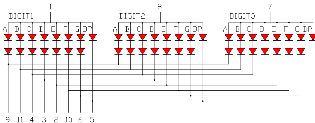
□ OPS-T8010LR-GW (Common Anode)
